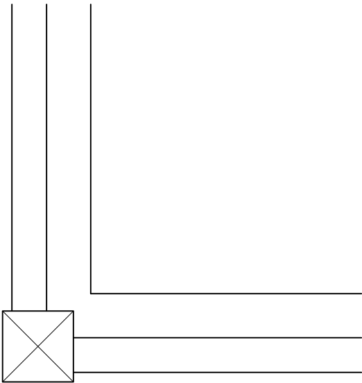
HÖRNLIST 45x45 MM RÅR 6 MM UTANFÖR PANELEN
